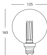
G125 E27 Globe id_nr 06-8622011
