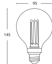
G95 E27 Globe id_nr 06-8622012
