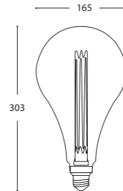
S165 E27 Drop id_nr 06-8622040
