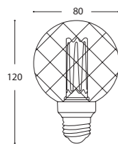
G80 E27 Mini Globe id_nr 06-8622013
